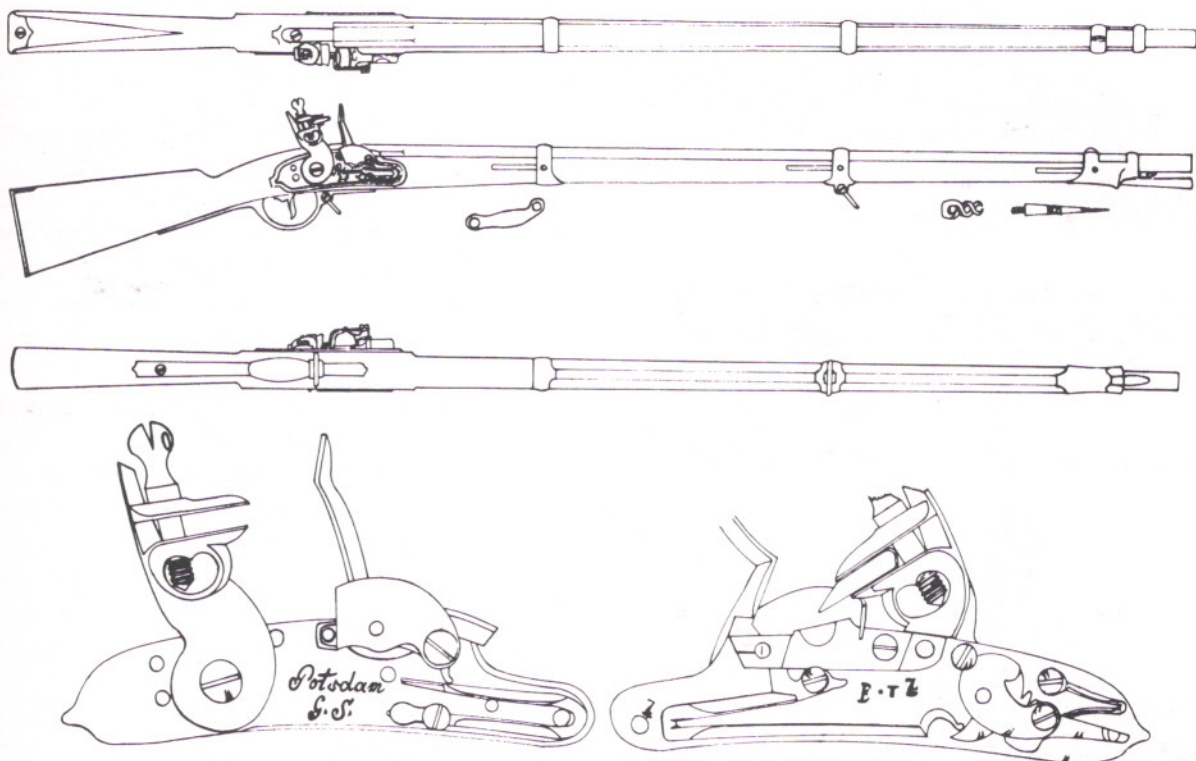
Infanterie-Gewehr M/1809 (sog. Neupreußisches Gewehr)
