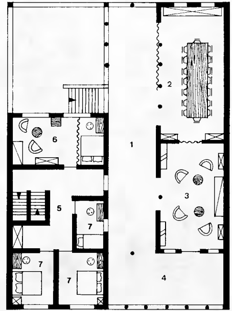
Obergeschoß (O)
