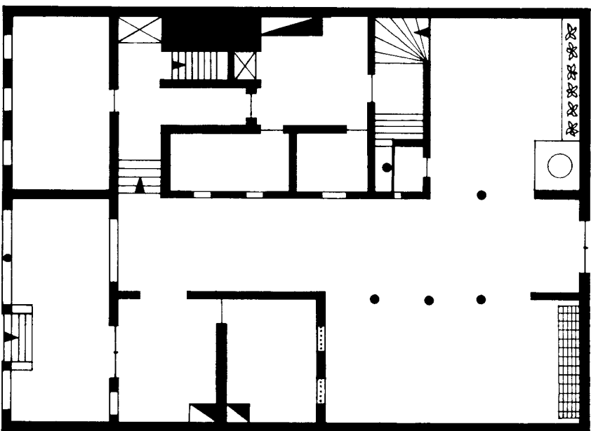
Erdgeschoß (E) 2 Schritt
