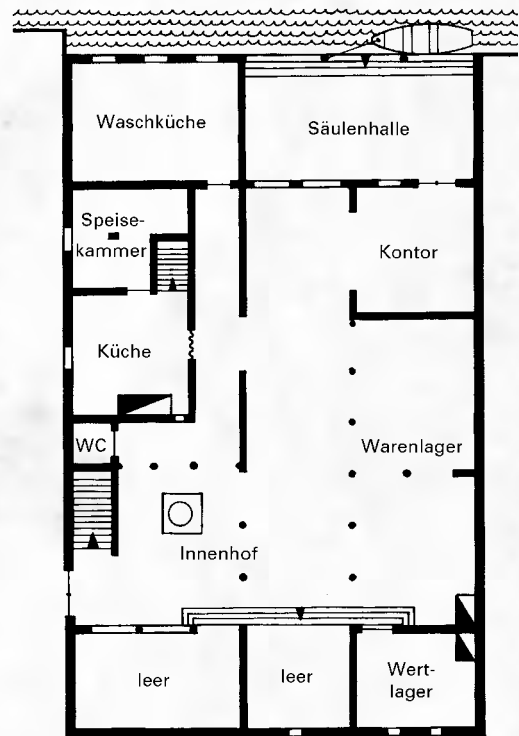
Untergeschoß
