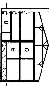
Querschnitt 4 Schritt
